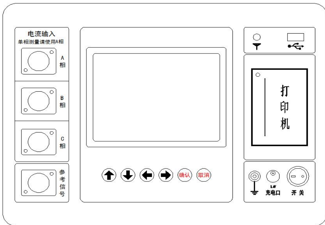
图 3 主机面板
