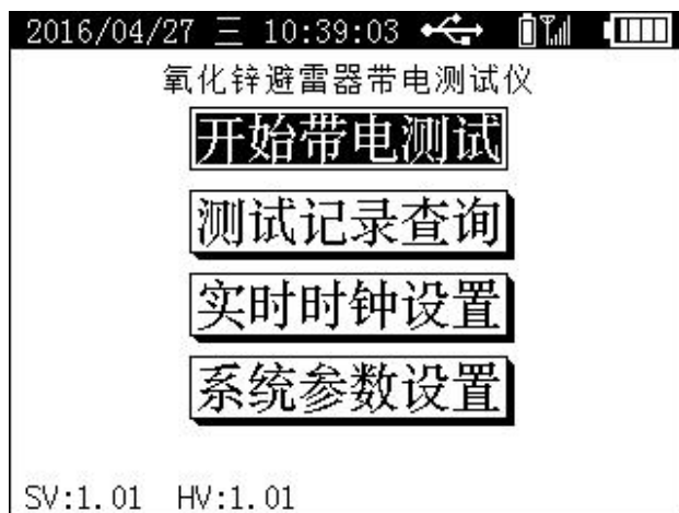
图7 主菜单
