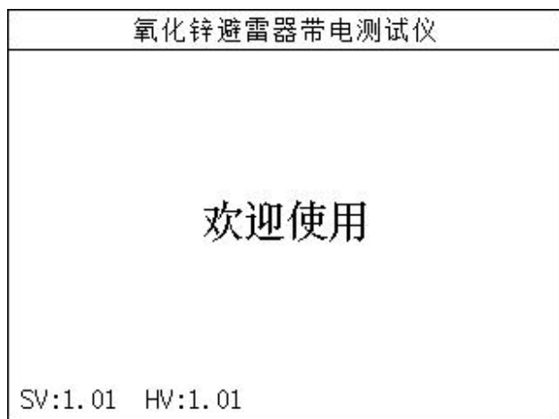
图6 开机屏幕
