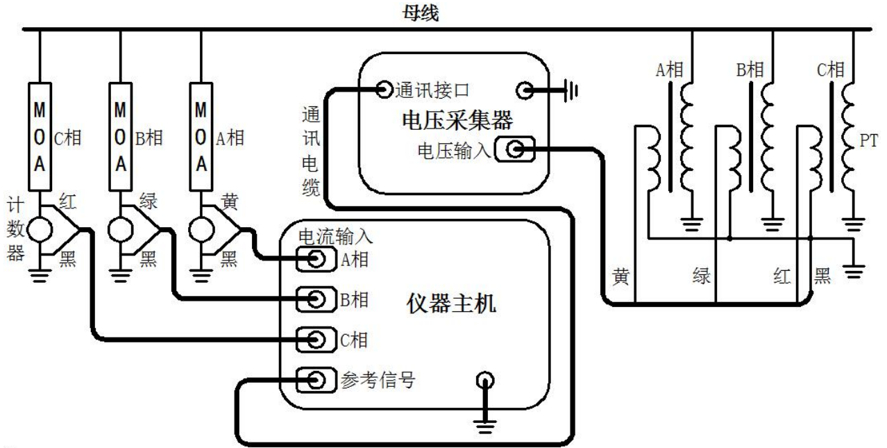
图 18 有线测试方式接线示意图（三相同步测量）
