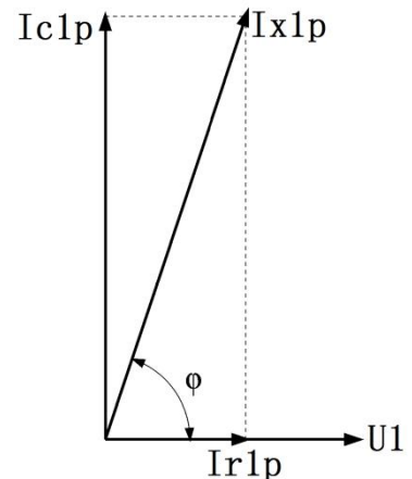
图 1 投影法
